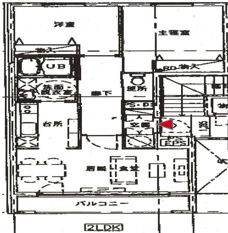
間取り
