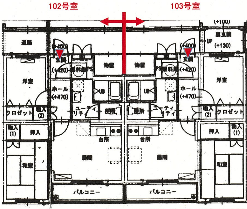
間取り
