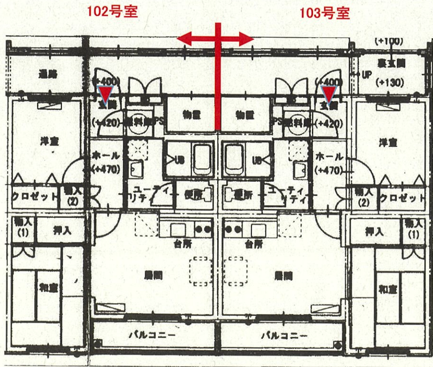
間取り
